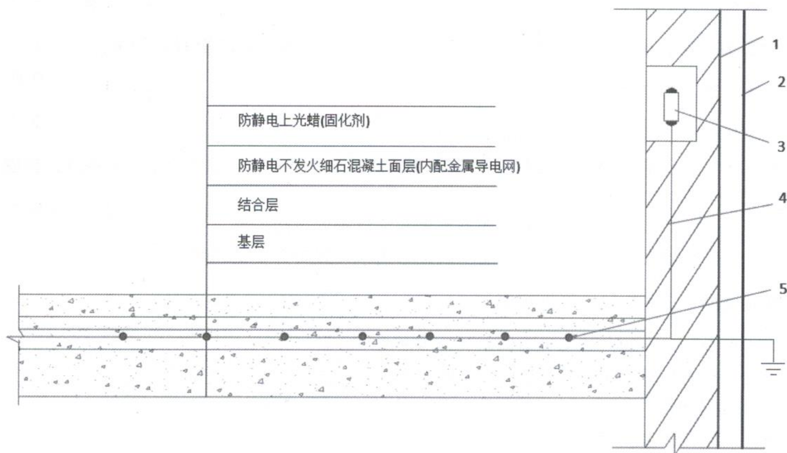
图4 安装接地系统及地坪构造示意图
