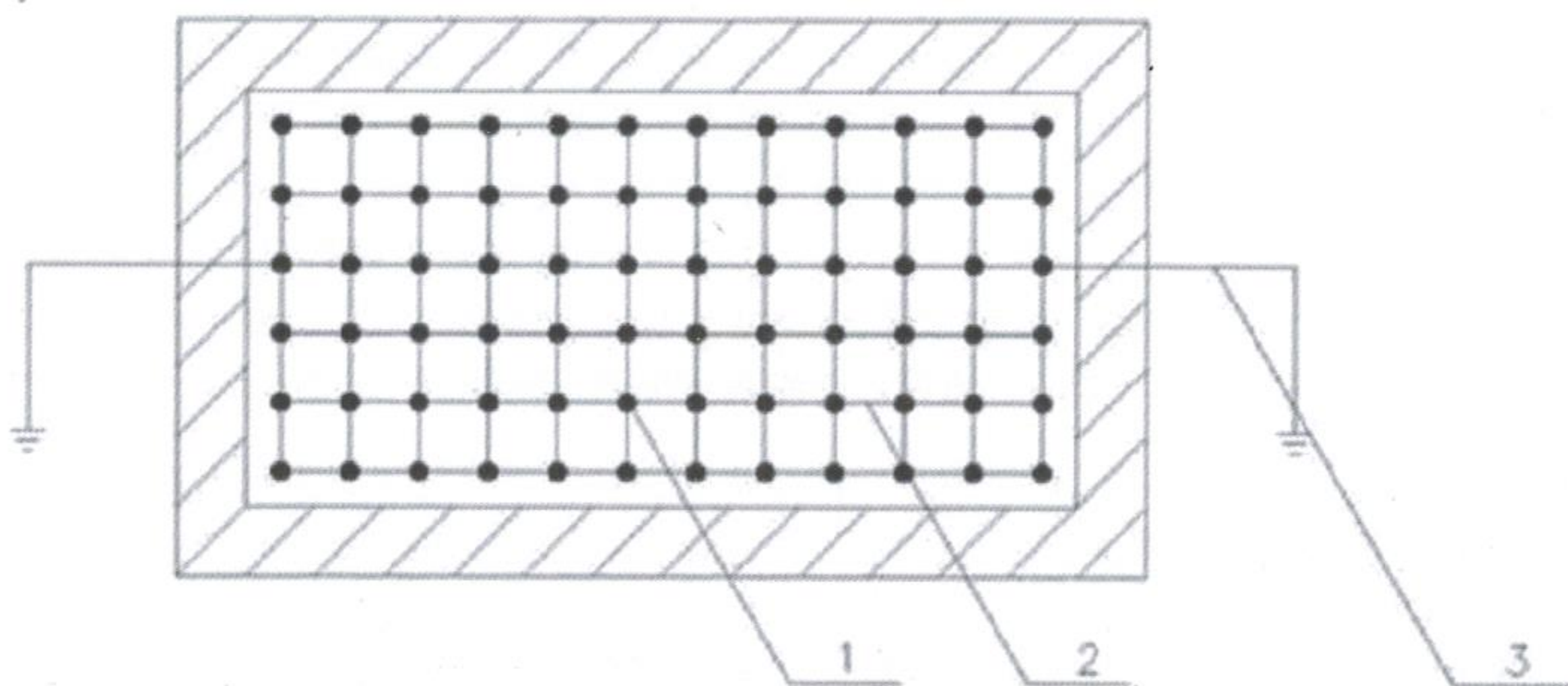
图 1 方阵形防静电接地网示意图
