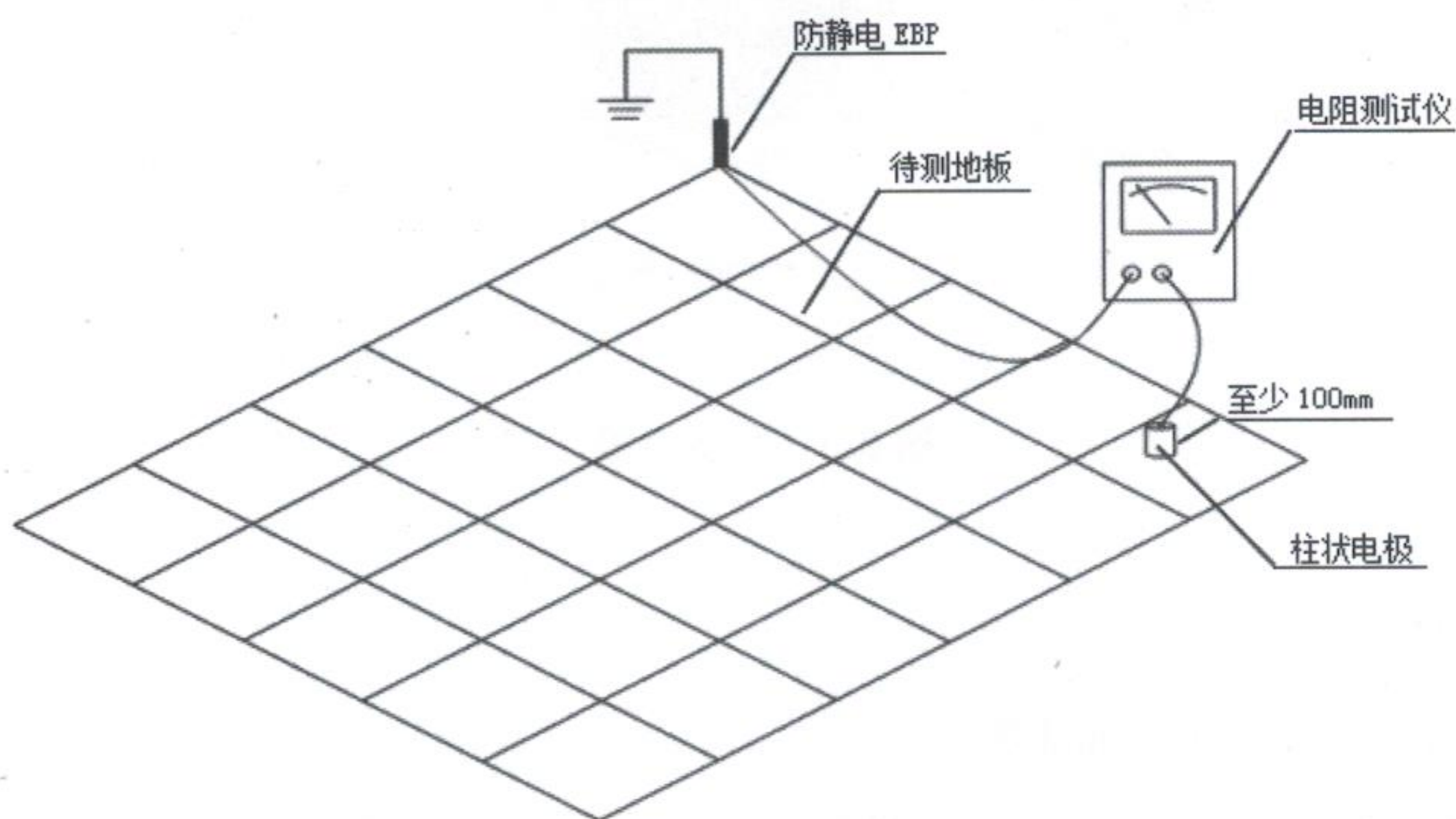
图 B.3 对地电阻测试方法示意图
