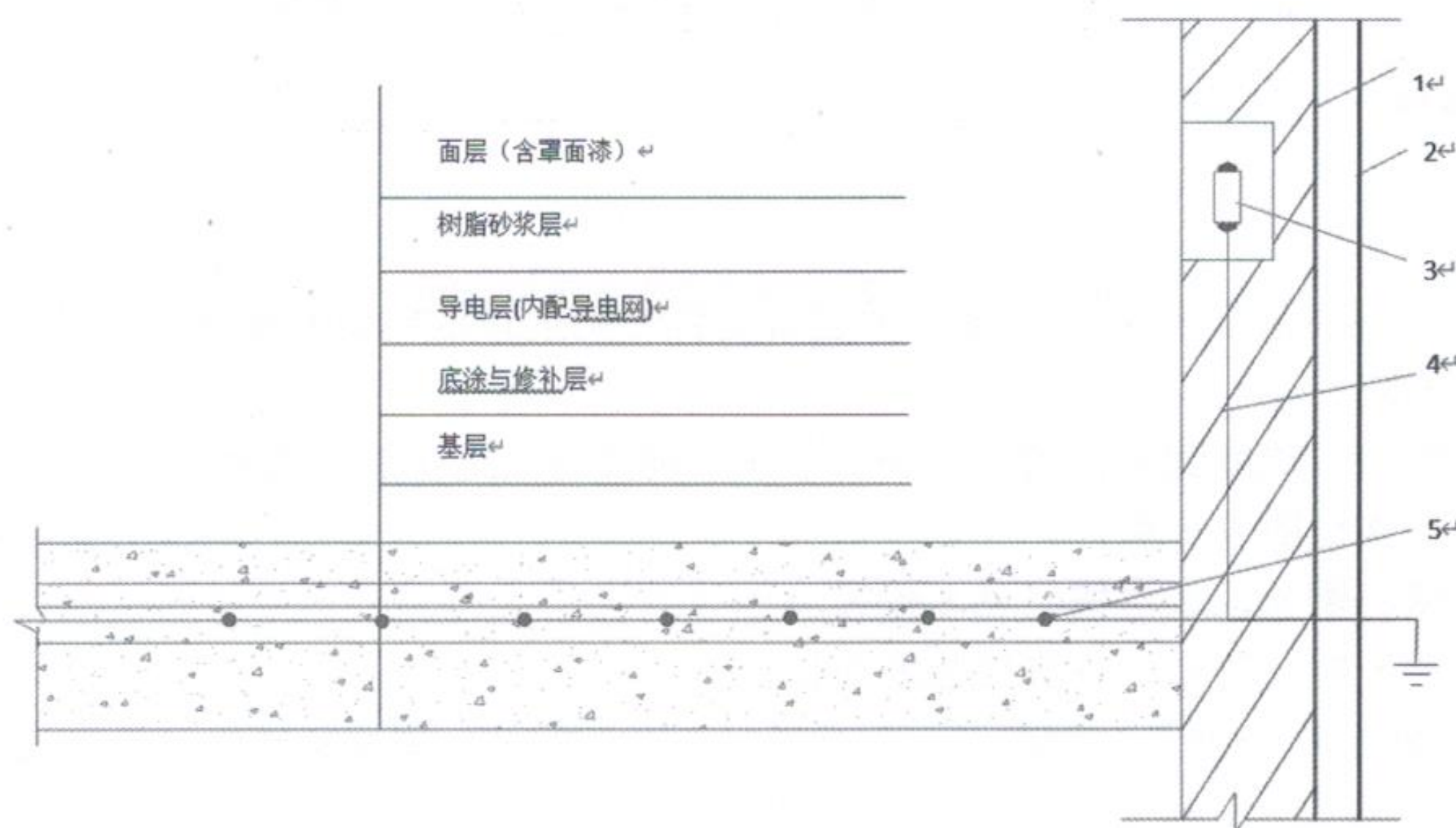
图8 安装接地系统及地坪构造示意图
