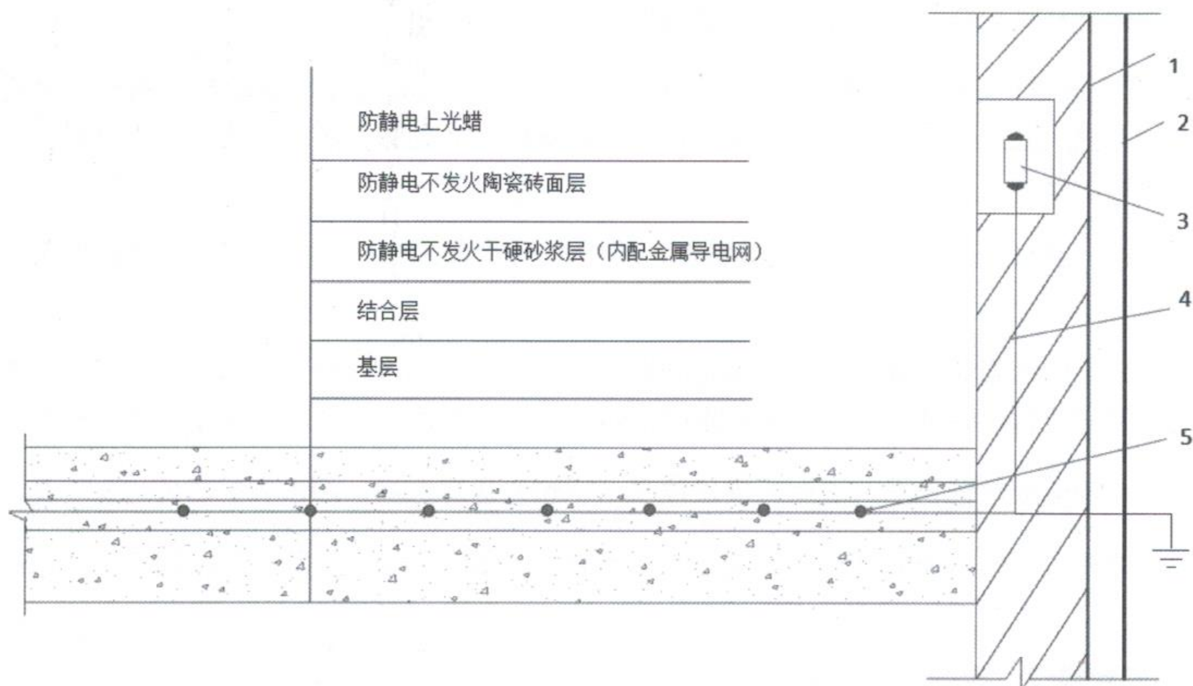
图7 接地系统与地坪构造示意图
