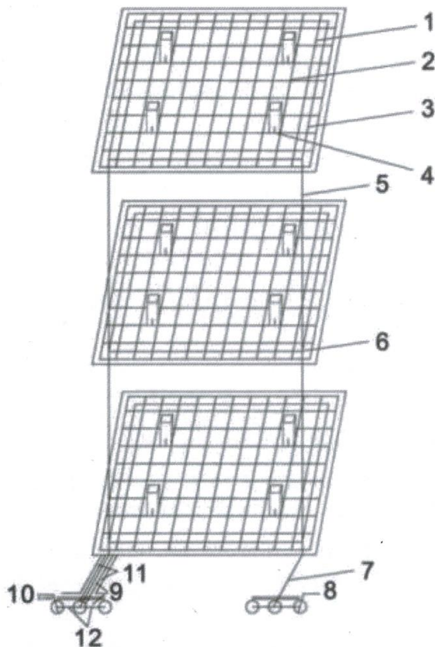
图10 防静电独立接地系统示意图
