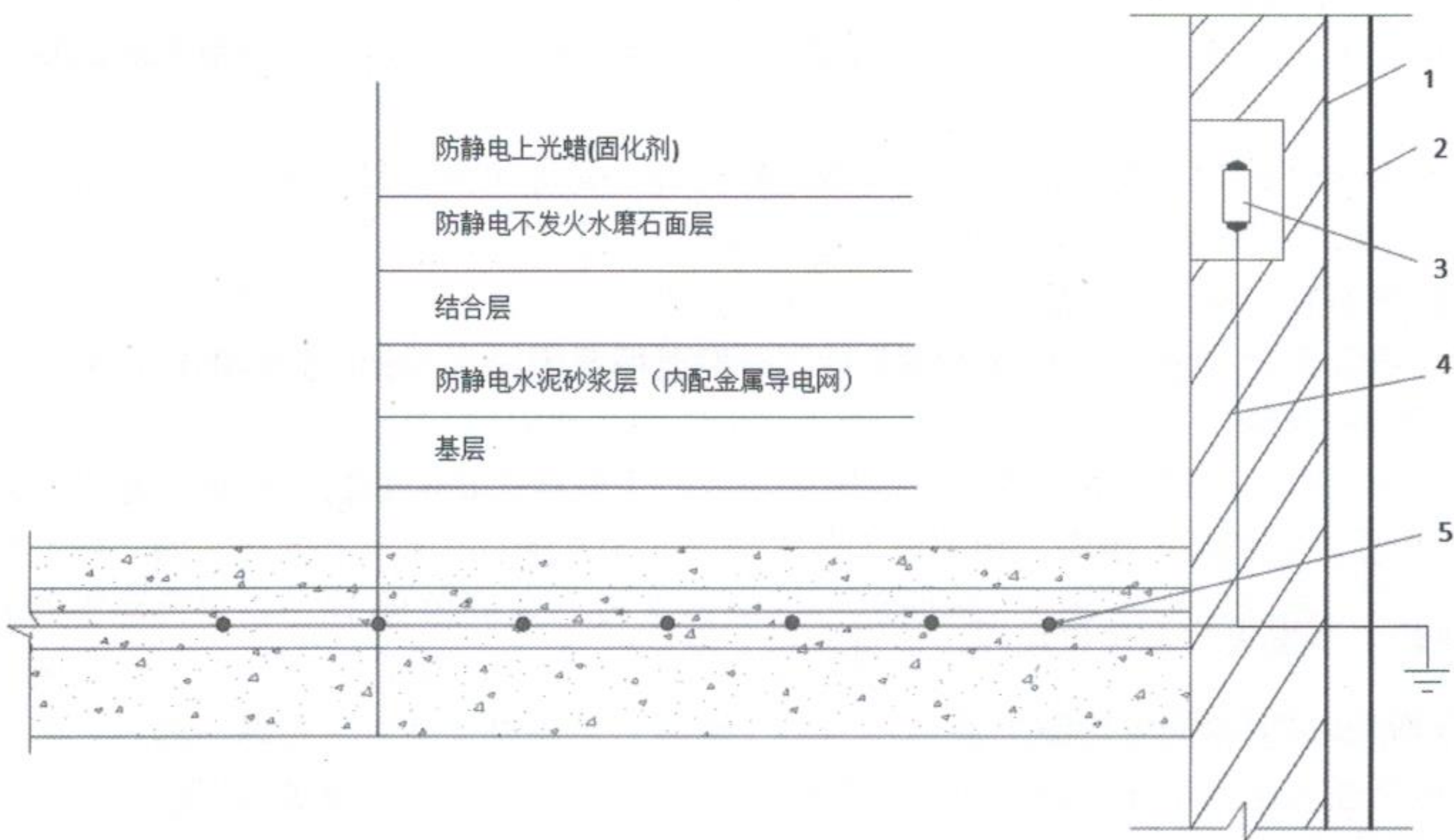
图 5 接地系统及地坪构造示意图
